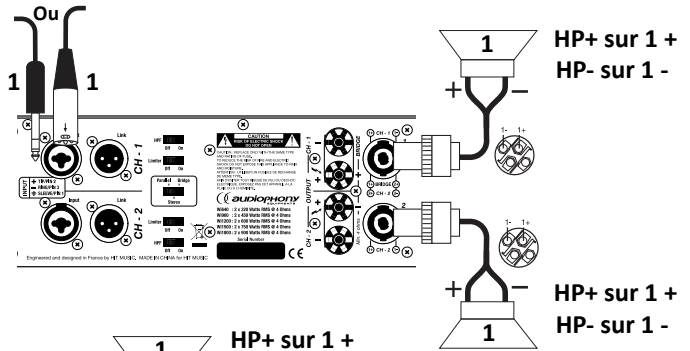
Mode parallèle normal
