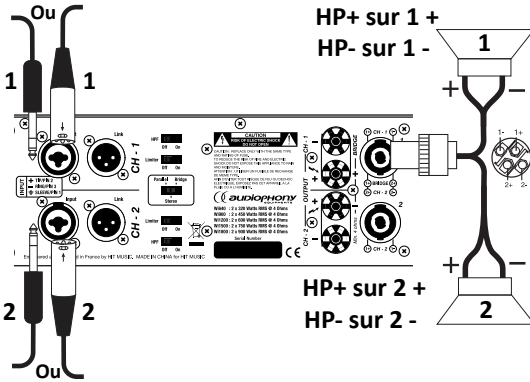
Mode Stéréo sur une seule sortie
