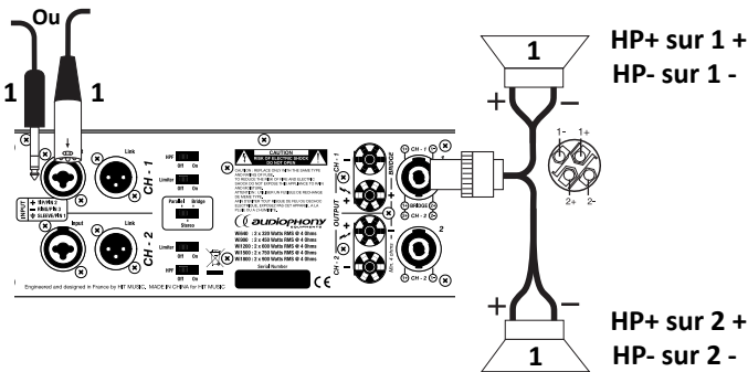
Mode parallèle sur une seule sortie
